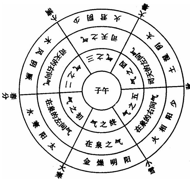
子午年司天在泉左右间气图
