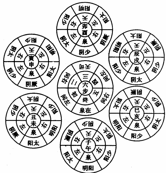
司天在泉左右间气位置图
